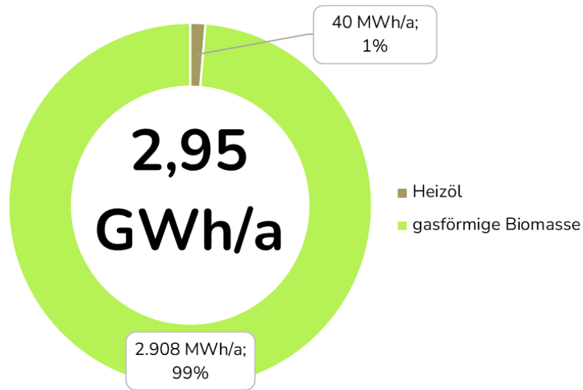
Abbildung 23: Jährlicher Endenergieverbrauch leitungsgebundener Wärme nach Energieträger (Veröffentlichung nach WPG, Anlage 2, I.)
