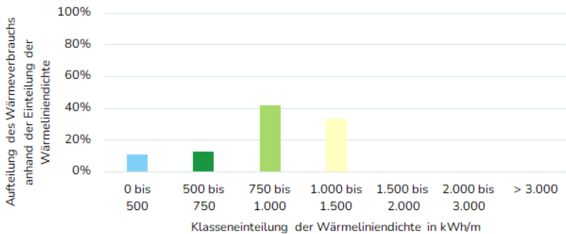
Anteile am Wärmeverbrauch - Thansüß
