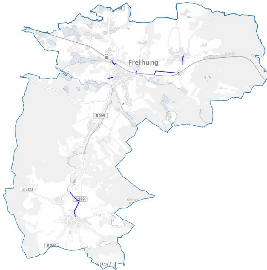
Abbildung 39: Abwassernetz gefiltert nach Abschnitten mit Höhe und Breite größer 800 mm (Veröffentlichung nach WPG, Anlage 2, II.)
