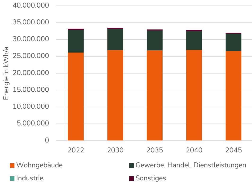
Abbildung 58: Wärmeverbrauch nach Sektoren in den Stützjahren (Veröffentlichung nach WPG, Anlage 2, III.)
