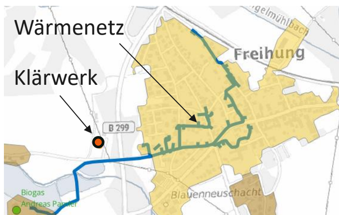
Abbildung 41: Kläranlagenstandort mit potenziell zu versorgenden Quartieren (Veröffentlichung nach WPG, Anlage 2, II.)
