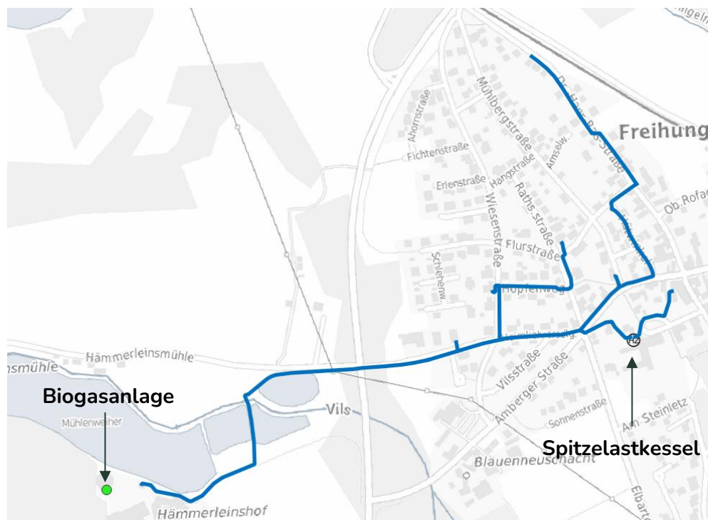
Abbildung 9: Wärmenetz Freihung (Veröffentlichung nach WPG, Anlage 2, I.)
