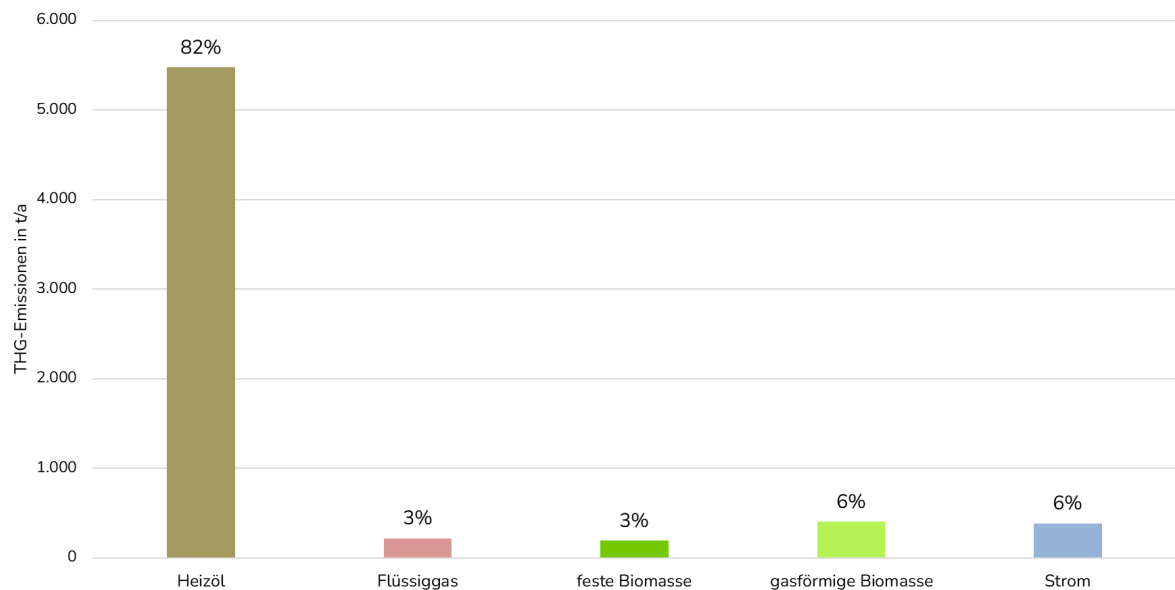
Abbildung 19: Treibhausgasemissionen nach Energieträger (Veröffentlichung nach WPG, Anlage 2, I.)
