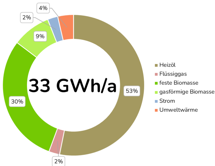
Abbildung 16: Endenergie im Wärmesektor
