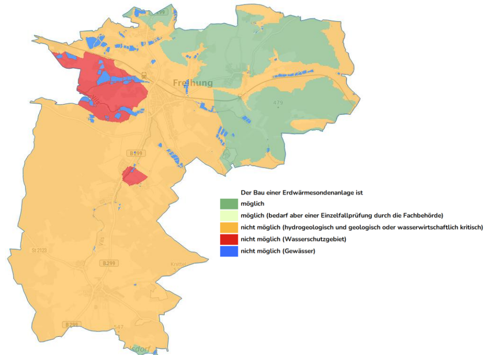
Abbildung 36: Potenziale für Erdwärmesonden (Veröffentlichung nach WPG, Anlage 2, II.) [Datenquelle: Bayerisches Landesamt für Umwelt, www.ifu.bayern.de ]
