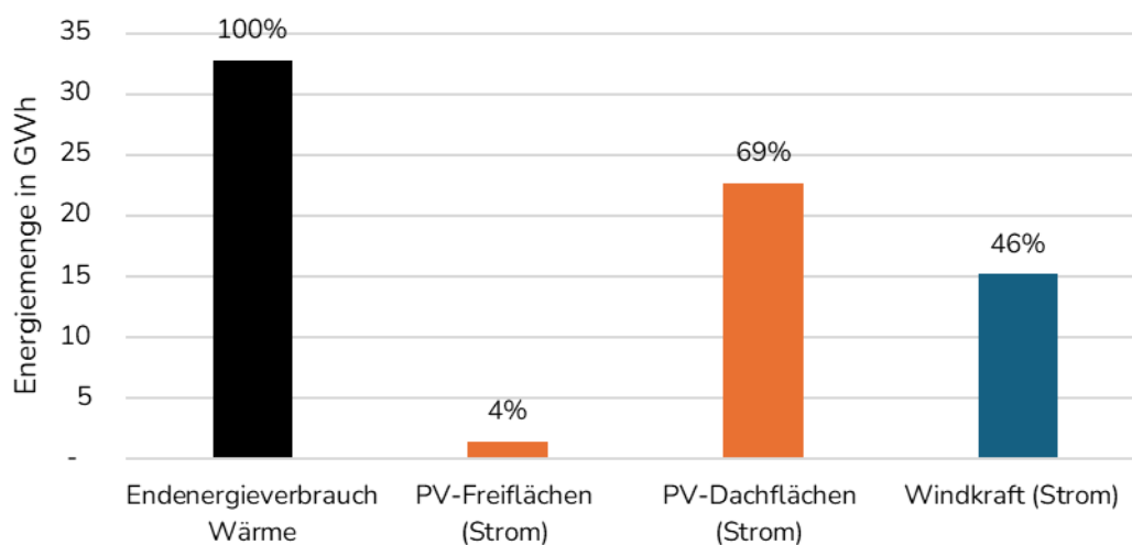
Abbildung 33: Energiemengen aus erneuerbaren Energie-Potenzialen im Vergleich zum gesamten Endenergieverbrauch Wärme von Freihung
