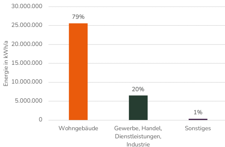
Abbildung 20: Wärmeverbrauch nach Sektoren (Veröffentlichung nach WPG, Anlage 2, I.)
